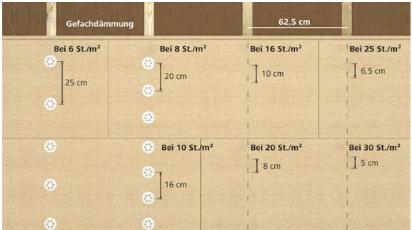
Beispiel: Sto-Weichfaserplatte M Nut und Feder, 130x60 cm, auf Holzständerwerk mit Achsmaß von 62,5 cm, mit Sto-Schraubdübel H 60 und Breitrückenklammern
